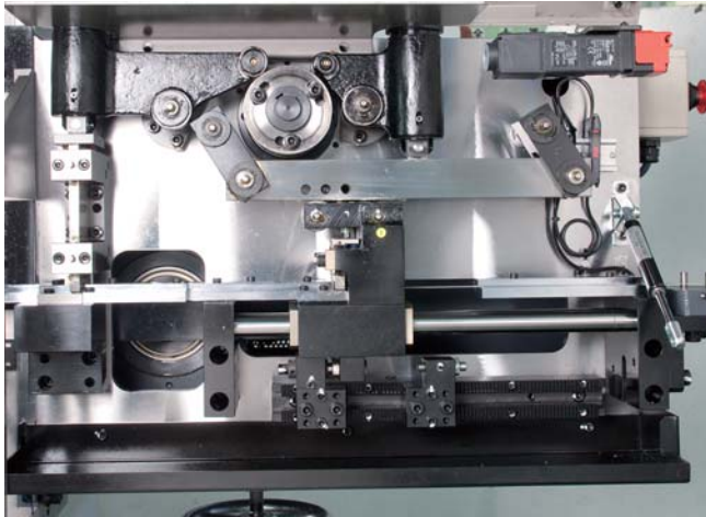
NC グリッパーフィードユニット NC gripper feed unit
