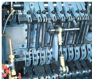
■パンチストリッパ&ストップリーフ装置 パンチから製品を管払いするのに使用します。
