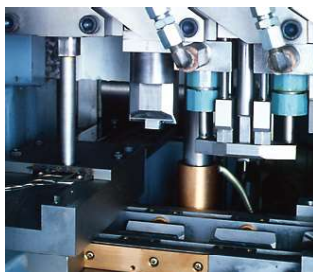
■ブランクホルダー装置 第2工程以降で、しわ押さえとしてブランクの絞り加工を確実にコントロールするのに使用します。
