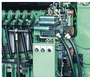
■NCオシレーティングフィーダー 2軸NC制御による材料のジグザグ送りに使用します。ブランク径、材料さん幅のキー入力をする と、ロール送り量、揺動量を自動演算します。
