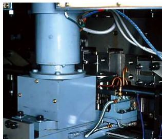
■スレッドローリング装置 トランスファープレスの右側又は中間部に取付けられ、ねじ成形、ローリングカット、ピーディング加工に使用します。
