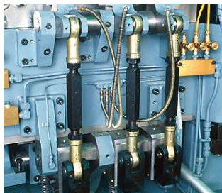
■クロスモーション装置 製品の横方向（前、後、左、右）からのピアシング、スロットング、フォーミング加工に使用します。
